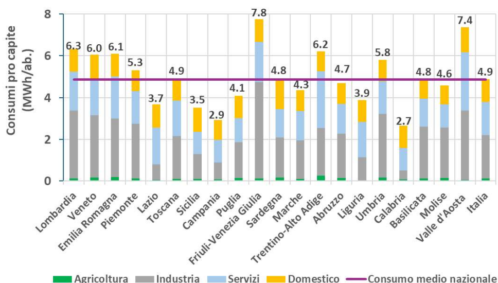
Figura 2.14 – Consumi elettrici pro capite per settore (2023); le etichette si riferiscono ai consumi totali pro capite.
