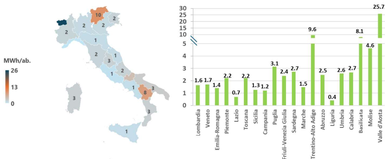
Figura 2.8 – Mappa regionale della produzione elettrica lorda per abitante da fonti rinnovabili al netto dei pompaggi e degli accumuli stand alone (2023).
