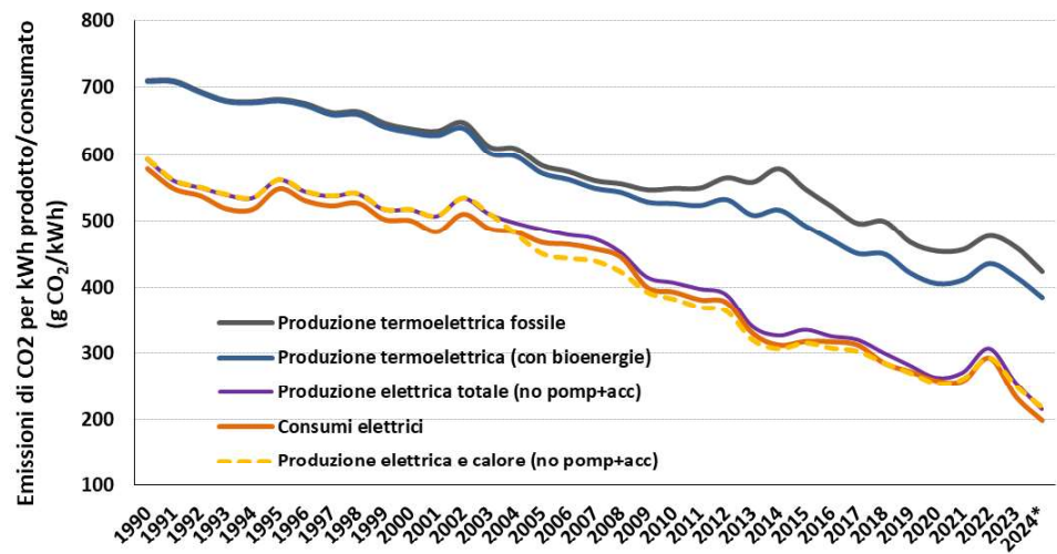
Figura 1.11 – Andamento dei fattori di emissione nel settore elettrico.
