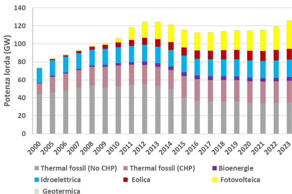
Figura 1.5 – Potenza efficiente lorda.
