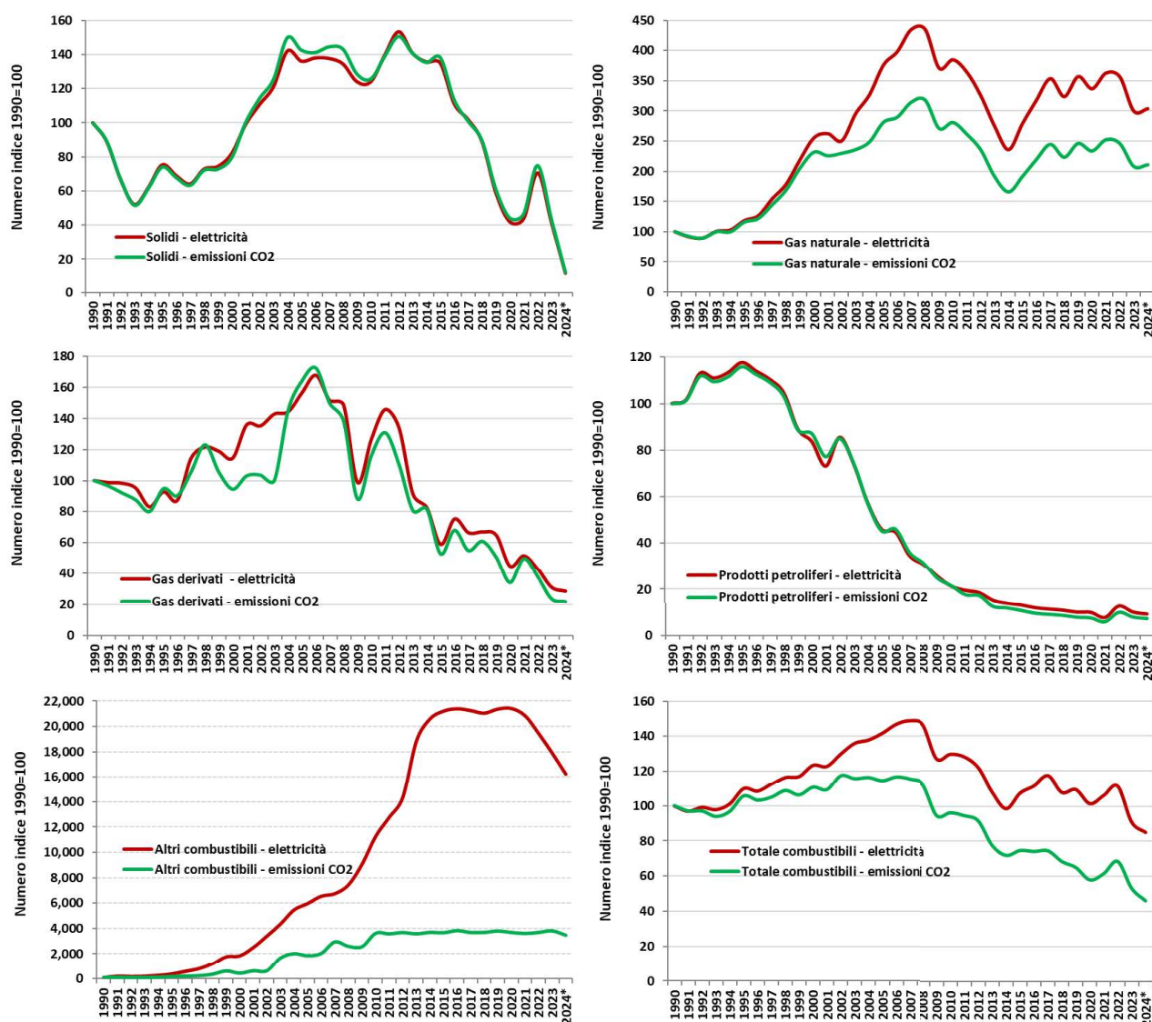
Figura 1.8 – Variazione annuale rispetto al 1990 della produzione termoelettrica e delle emissioni di CO 2 per combustibile (1990=100).
