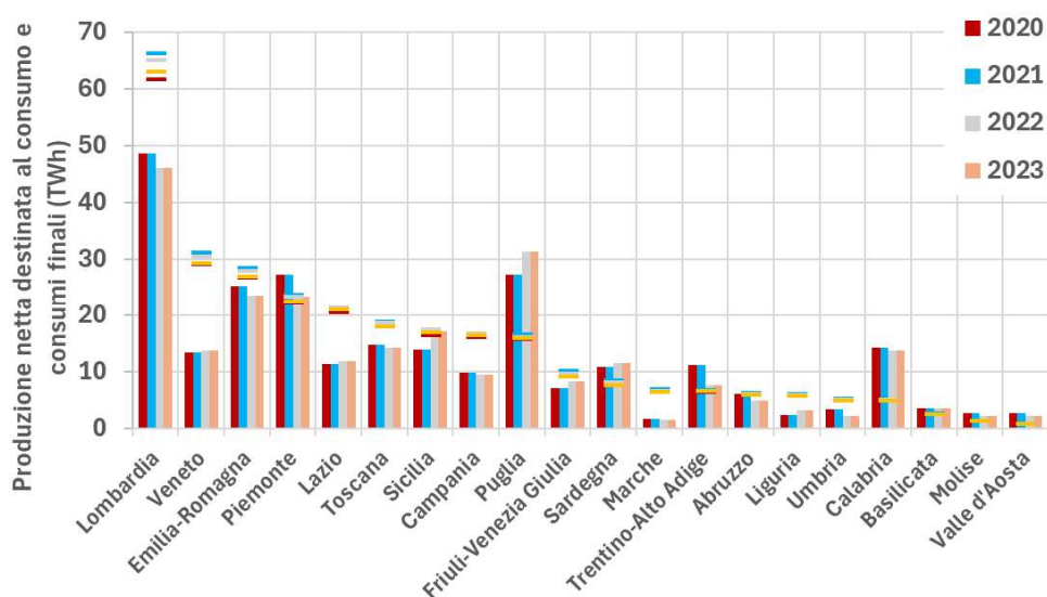
Figura 2.15 – Confronto tra consumi finali di energia elettrica (linee) e produzione interna destinata al consumo al netto delle perdite di rete (barre).
