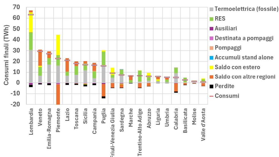
Figura 2.20 – Produzione elettrica destinata al consumo al netto delle perdite di rete e saldo import-export con estero e con altre regioni (2023).
