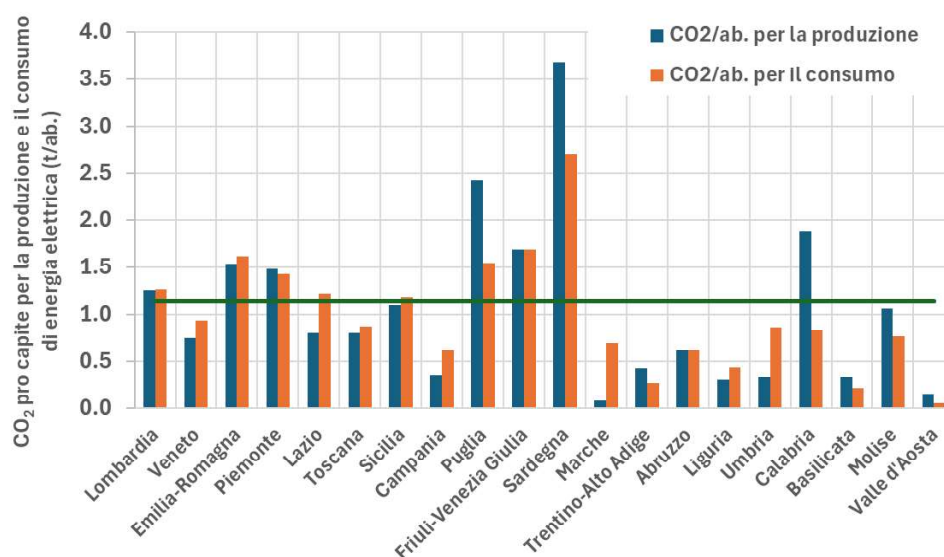
Figura 3.12 – Emissioni di CO 2 pro capite per la produzione e il consumo di energia elettrica ripartendo la quota di energia elettrica importata nei due macro-compartmenti individuati (2023).
