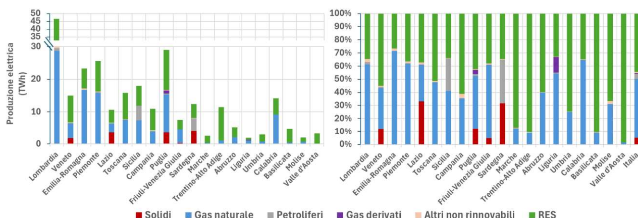
Figura 2.10 – Produzione elettrica lorda per fonte (2023).
