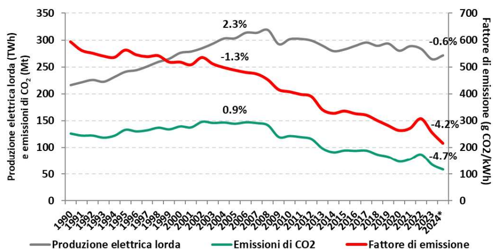
Figura 1.10 – Andamento della produzione elettrica lorda, emissioni di CO 2 (asse a sinistra) e fattori de emissione (asse a destra). Le etichette si riferiscono al tasso di variazione media annuale, dal 1990 al 2005 e dal 2005 al 2024.
