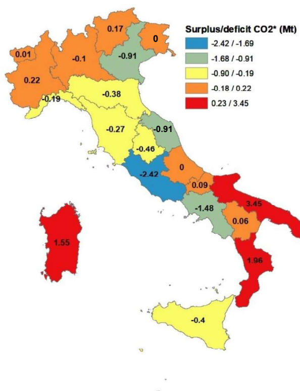
Figura 3.15 – Mappa regionale del surplus/deficit della produzione elettrica e delle emissioni di CO 2 rispetto ai consumi interni del 2023.
