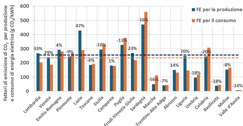
Figura 3.5 – Fattori di emissione di CO 2 per la produzione e il consumo di energia elettrica. Con le linee tratteggiate è rappresentate le medie nazionale dei due fattori di emissione (2023). Le etichette si riferiscono al delta percentuale tra fattore di emissione per la produzione e fattore di emissione per il consumo.
