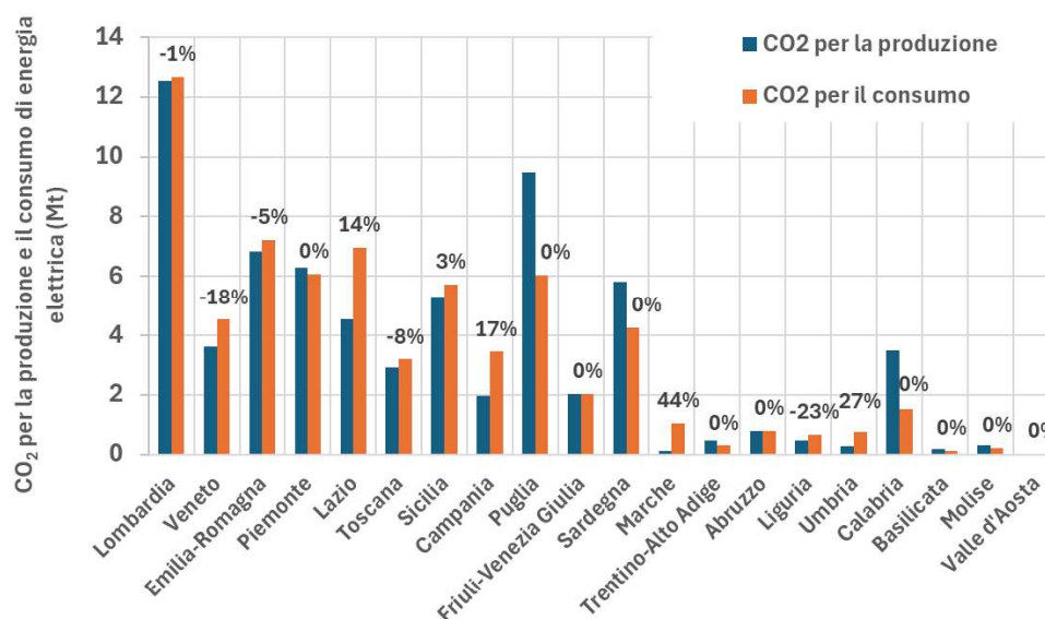
Figura 3.11 – Emissioni di CO 2 per la produzione e il consumo di energia elettrica ripartendo la quota di energia elettrica importata nei due macro-compartmenti individuati (2023). Le etichette si riferiscono alla variazione della CO 2 emessa per i consumi rispetto al dato riportato in Figura 3.3.
