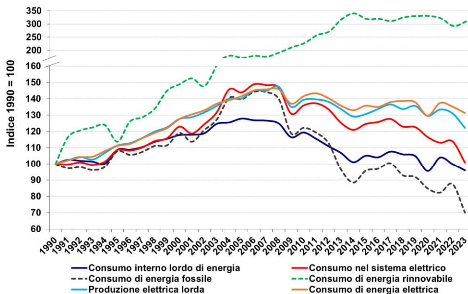
Figura 1.2 – Andamenti indicizzati del consumo interno lordo di energia, del consumo di energia nel settore elettrico per la produzione di elettricità e calore, della produzione e consumo di energia elettrica.
