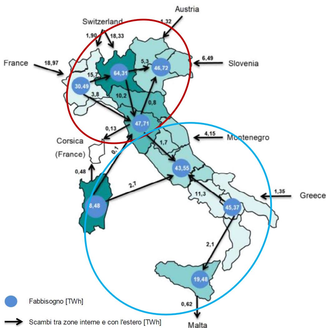
Figura 3.10 – Saldo dei movimenti fisici di energia nel 2023 (TERNA, 2024). Le ellissi circoscrivono i due macro-compartimenti considerati per la ripartizione della quota elettrica importata dall'estero.
