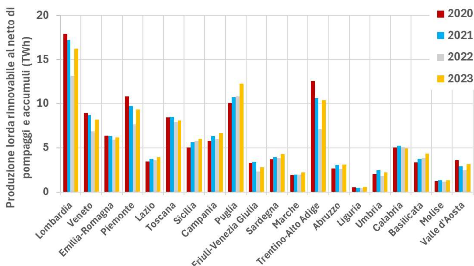
Figura 2.5 – Produzione elettrica lorda da energie rinnovabili al netto dei pompaggi e degli accumuli stand alone nelle regioni.
