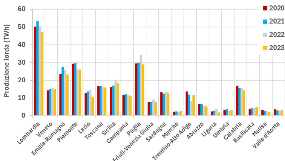
Figura 2.2 – Produzione elettrica lorda nelle regioni.
