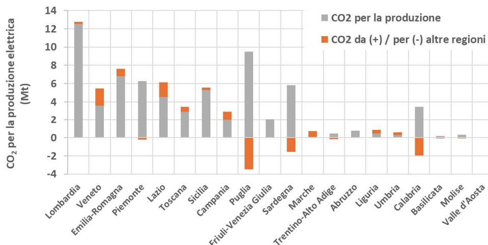
Figura 3.8 – Saldo import-export con estero e con altre regioni (2023).
