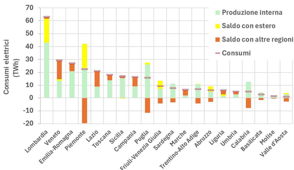
Figura 2.18 – Consumi elettrici delle regioni espressi in termini di produzione interna (energia destinata al consumo al netto delle perdite di rete) e saldo import-export con l'estero o con altre regioni (2023).
