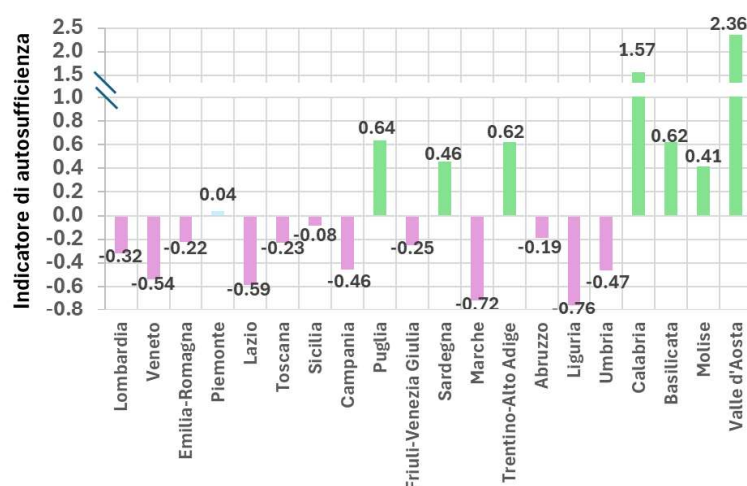
Figura 2.17 – Indicatore di autosufficienza della produzione netta regionale destinata al consumo per soddisfare il fabbisogno elettrico della regione.
