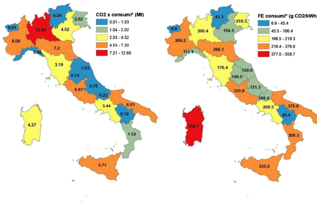
Figura 3.14 – Mappe regionali delle emissioni di CO 2 e dei fattori di emissione per i consumi (2023) ripartendo la quota di energia elettrica importata nei due macro-compartimenti individuati.
