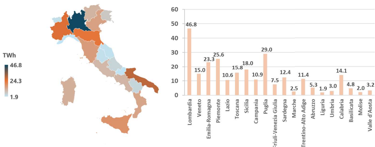
Figura 2.3 – Mappa regionale della produzione elettrica lorda al netto dei pompaggi e degli accumuli stand alone (2023).
