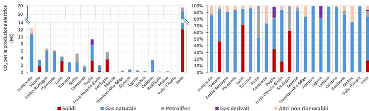
Figura 3.6 – Emissione di CO 2 per la produzione elettrica per tipologia di combustibile (2023).
