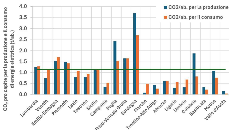
Figura 3.4 – Emissioni di CO 2 pro capite per la produzione e il consumo di energia elettrica (2023).
