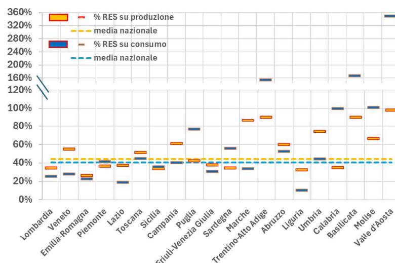
Figura 2.23 – Quota di energia elettrica rinnovabile lorda prodotta su produzione totale e consumi elettrici (2023).
