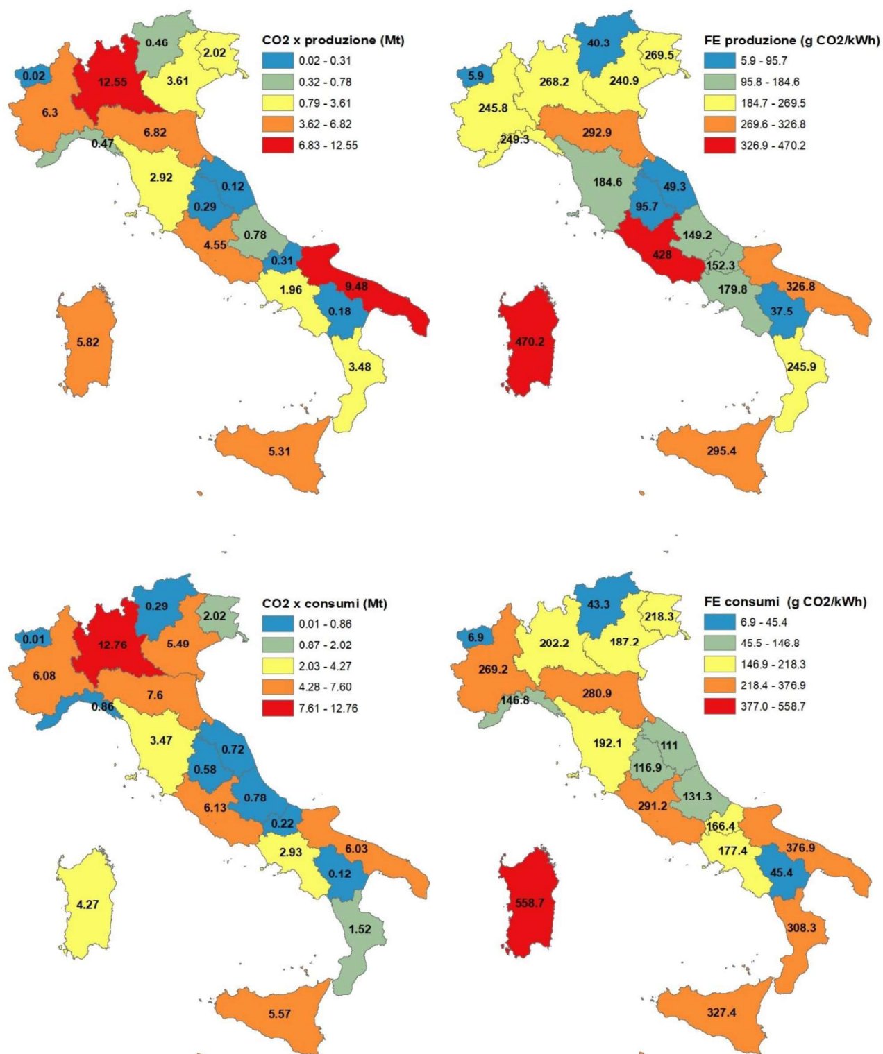
Figura 3.7 – Mappe regionali delle emissioni di CO 2 e dei fattori di emissione per la produzione elettrica e per i consumi (2023).
