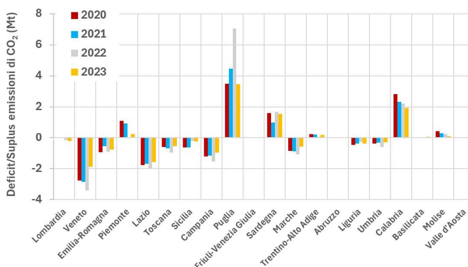
Figura 3.2 – Deficit/Surplus di CO 2 emessa in fase di produzione rispetto al consumo di energia elettrica.
