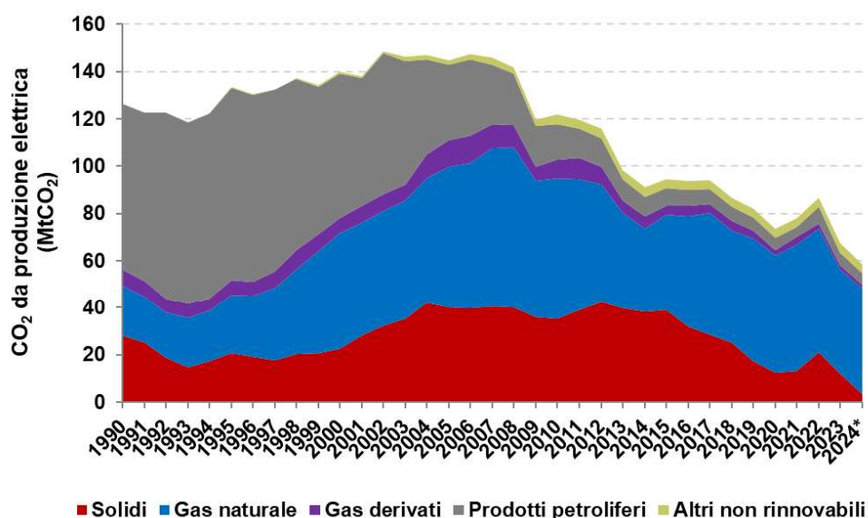
Figura 1.7 – Quota di emissioni di CO 2 per fonte.
