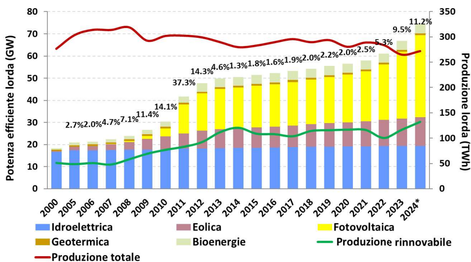
Figura 1.6 – Potenza efficiente lorda degli impianti rinnovabili (asse a sinistra) e produzione elettrica lorda (asse a destra). La percentuale si riferisce al tasso medio annuo di variazione della potenza totale.
