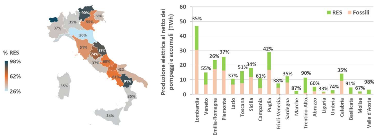
Figura 2.9 – Mappa regionale della quota di produzione elettrica da fonti rinnovabili (2023). Il grafico a destra riporta la produzione elettrica lorda ripartita per quota fossile e rinnovabile. Le etichette si riferiscono alla quota rinnovabile rispetto alla produzione totale al netto dei pompaggi e degli accumuli stand alone.
