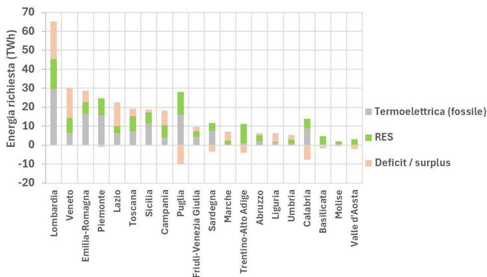
Figura 2.21 – Produzione elettrica destinata al consumo al netto delle perdite di rete e saldo import-export con estero e con altre regioni (2023).
