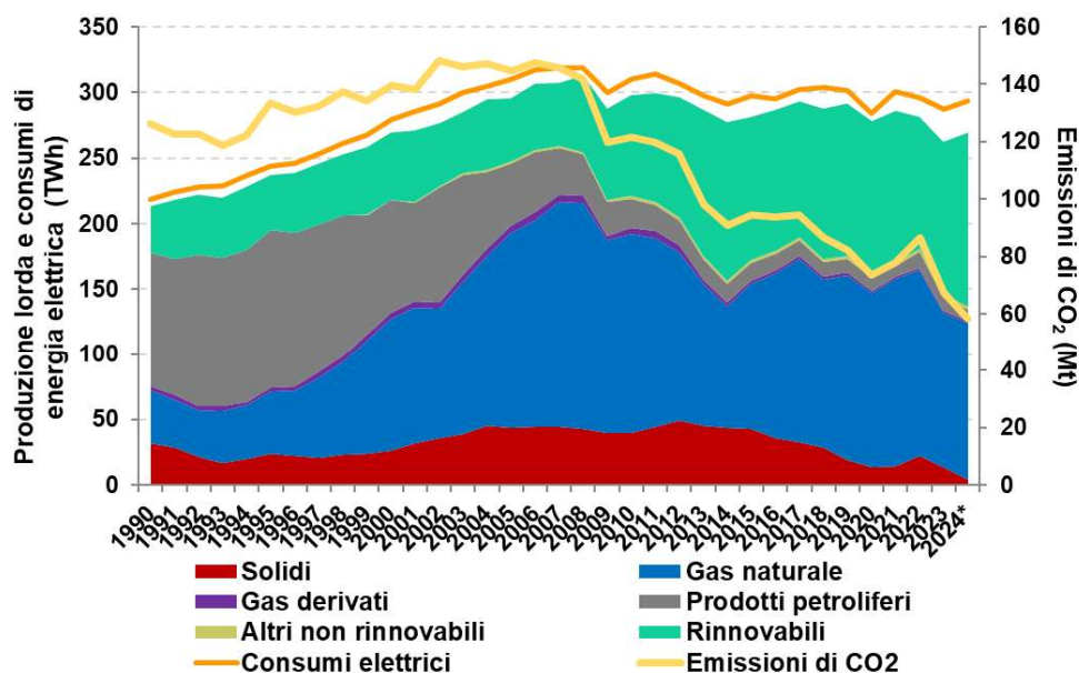
Figura 1.9 – Produzione lorda di energia elettrica per fonte, consumi elettrici e emissioni di CO 2 per la generazione elettrica.
