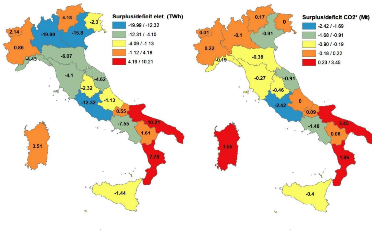
Figura 3.9 – Mappe regionali del surplus/deficit della produzione elettrica e delle emissioni di CO 2 rispetto ai consumi interni del 2023.
