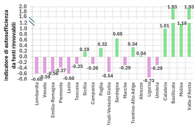
Figura 2.26 – Proiezioni al 2030 dell'indicatore di autosufficienza elettrica da fonti rinnovabili lorda rispetto ai consumi regionali.
