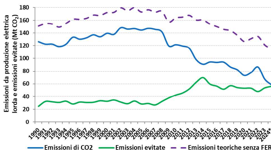
Figura 1.14 – Andamento delle emissioni di CO 2 dal settore elettrico e delle emissioni evitate.
