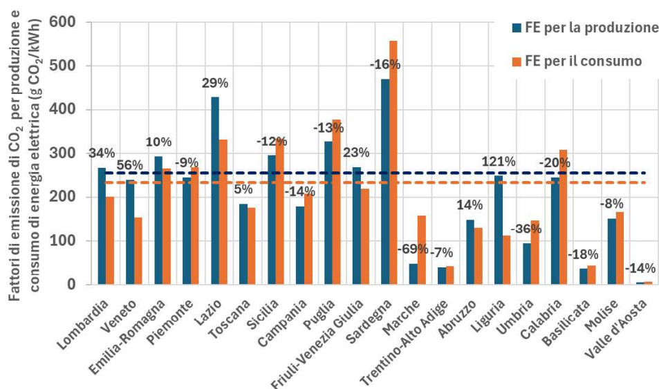
Figura 3.13 – Fattori di emissione di CO 2 per la produzione e il consumo di energia elettrica ripartendo la quota di energia elettrica importata nei due macro-compartmenti individuati. Con le linee tratteggiate è rappresentate le medie nazionale dei due fattori di emissione (2023). Le etichette si riferiscono al delta percentuale tra fattore di emissione per la produzione e fattore di emissione per il consumo.
